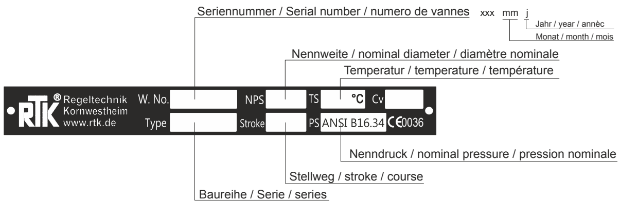
Bild 2/ Figure 2 : Typenschild nach ANSI auf Ventil / nameplate on valve acc. to ANSI
