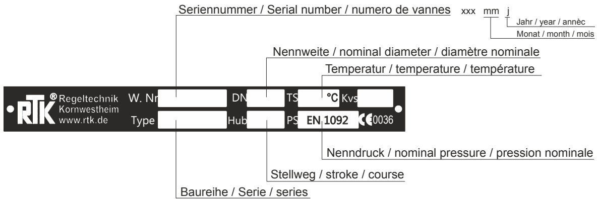
Bild 1/ Figure 1 : Typenschild nach DIN auf Ventil / nameplate on valve acc. to DIN
