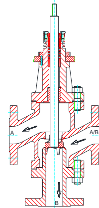
MV 5421 DN 80-250, PN 16-40
