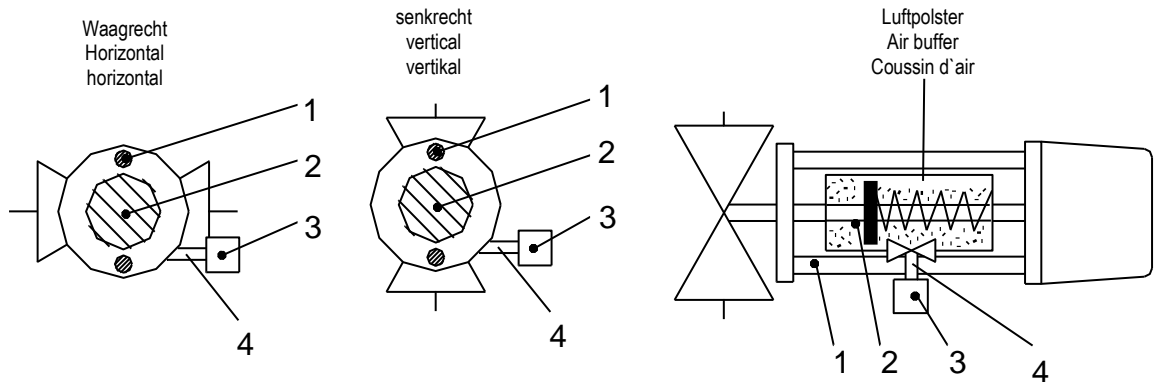
Bild 1 / figure 1 / photo 1: Einbau Schnellschlusseinrichtung waagerechter Einbau / mounting position emergency closing horizontally / position de montage horizontal
